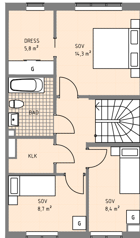
ÖVERVÅNING
