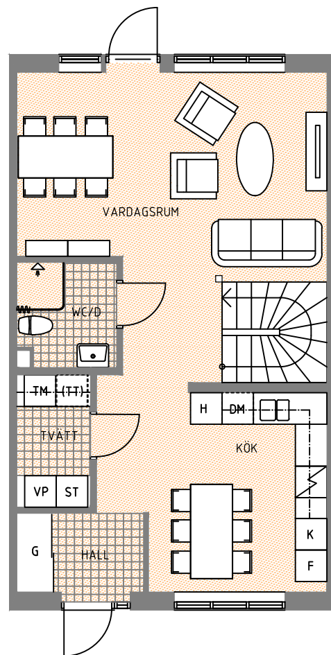
ENTRÉPLAN
