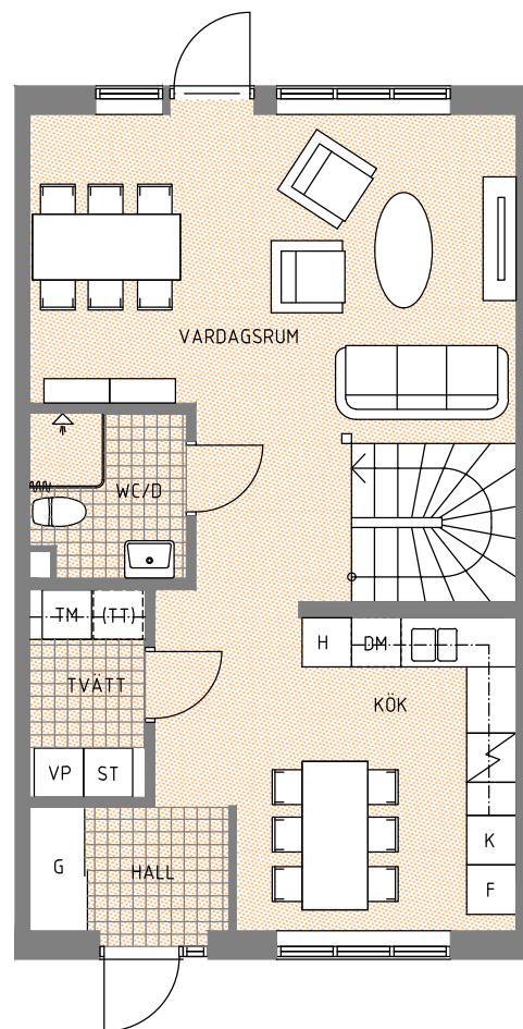
ENTRÉPLAN
