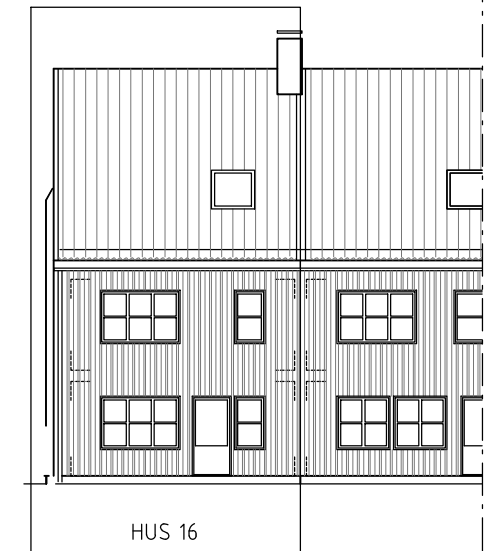
BAKSIDA SKALA 1:200
