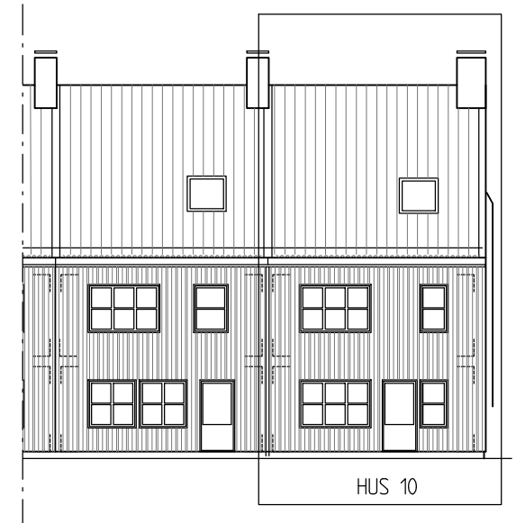
BAKSIDA SKALA 1200
